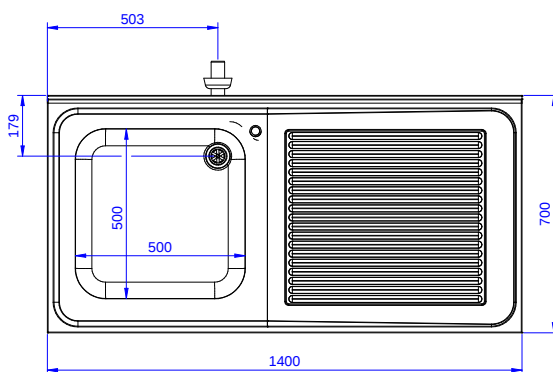
Boven aanzicht
