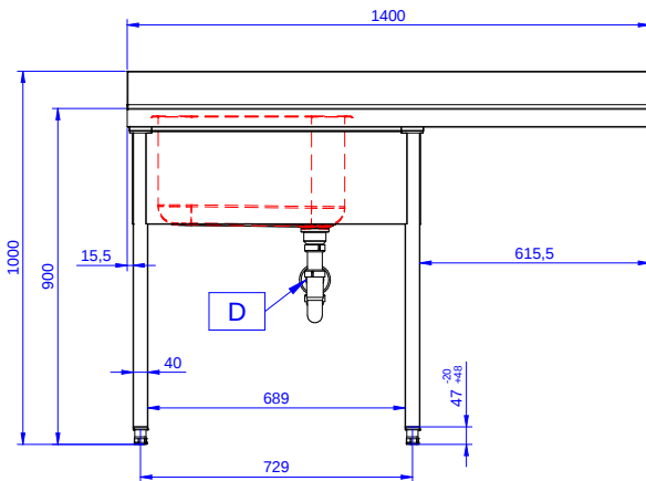
Zij aanzicht
